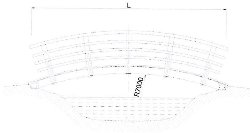
Rysunek 12. Przykładowa wizualizacja kładki dla pieszych nad ciekim wodnym.
