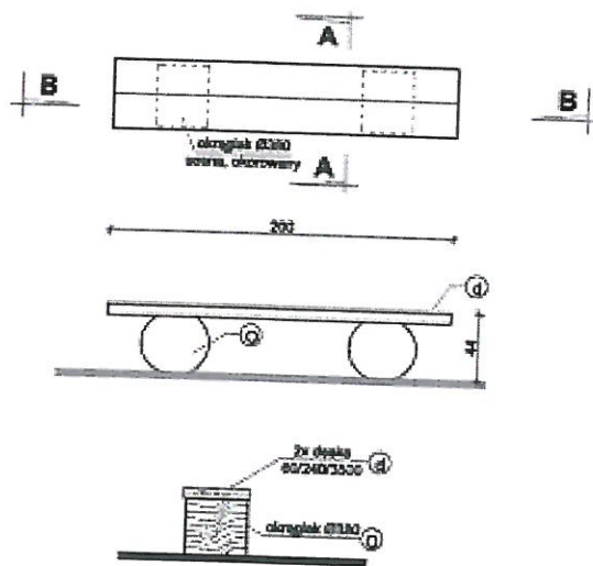
SIEDZISKO DOKOŁA OGNISKA
