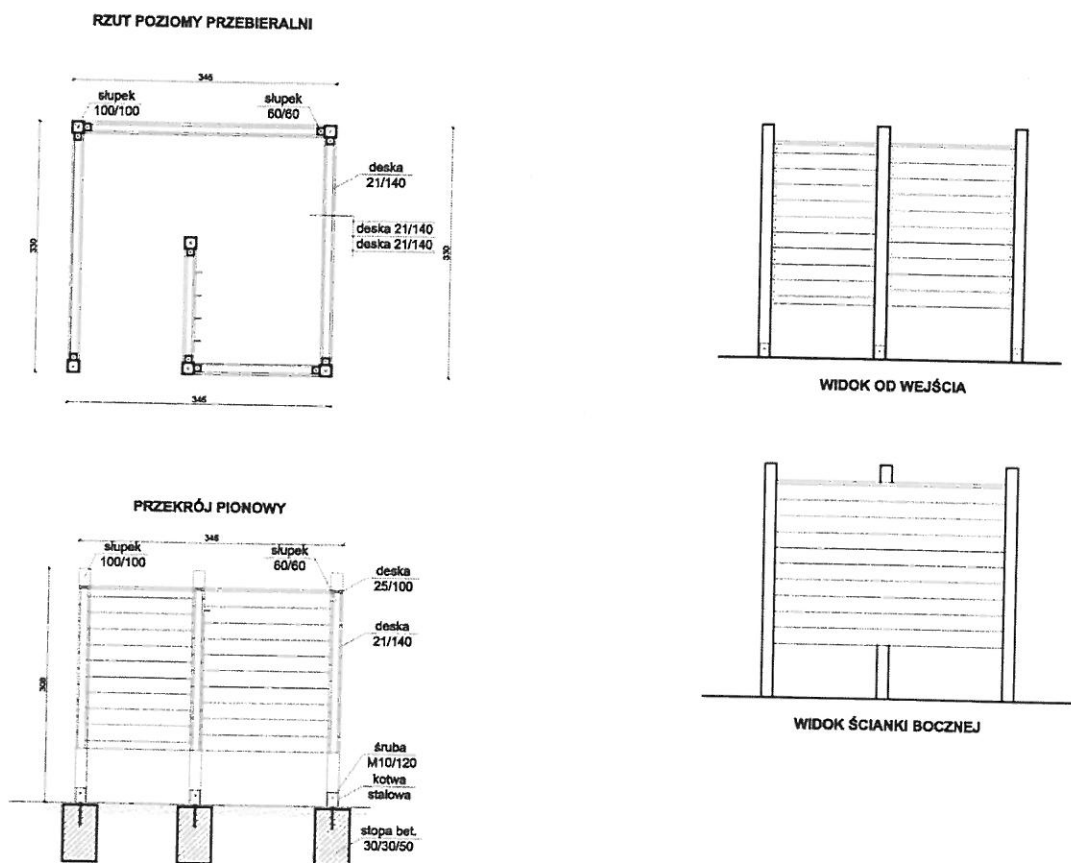
Rysunek 11. Przykładowa przebieralnia typu „ślimak”.
