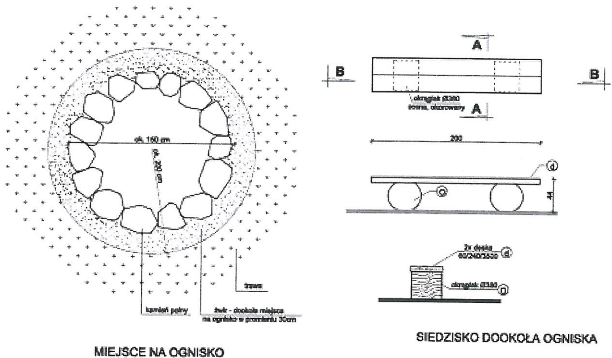
Rysunek 10. Przykładowe miejsce na ognisko.
