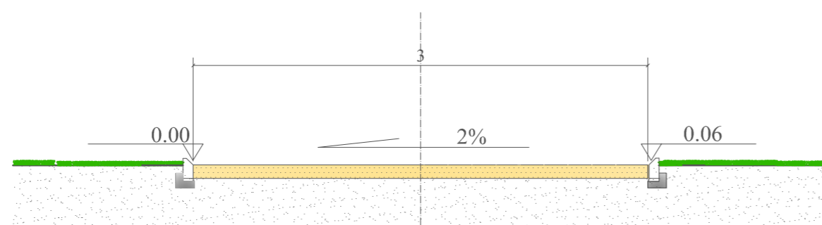
PROJEKTOWANE CIĄGI PIESZO-JEZDNE SKALA 1:20
