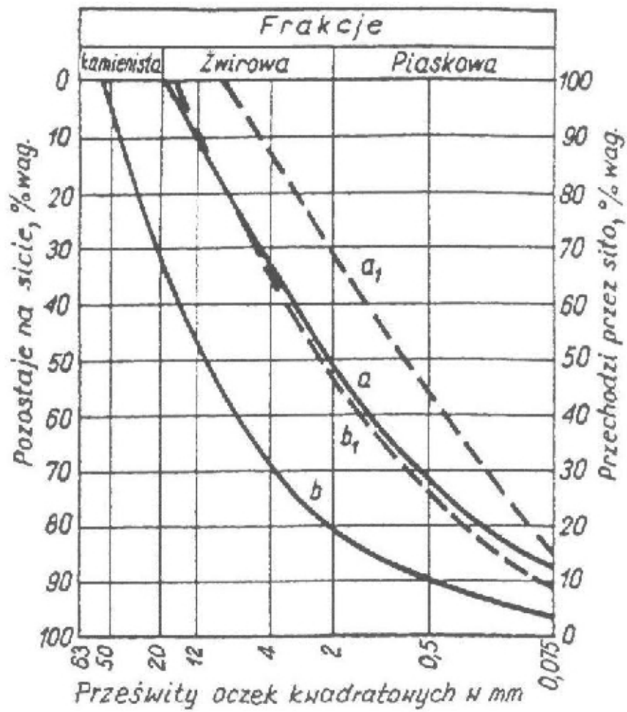
Rysunek 1. Obszar uziarnienia optymalnych mieszanek zwirowych
